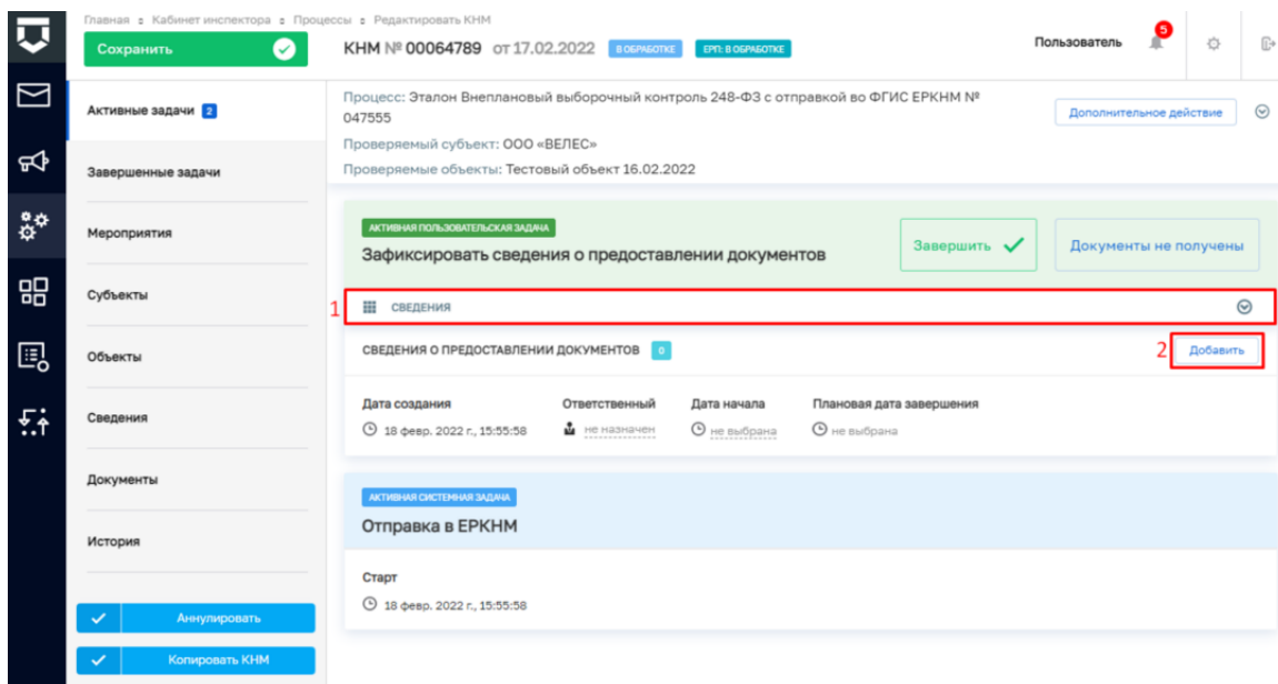
Рисунок 26. Работа с задачей "Зафиксировать сведения о предоставлении документов"
