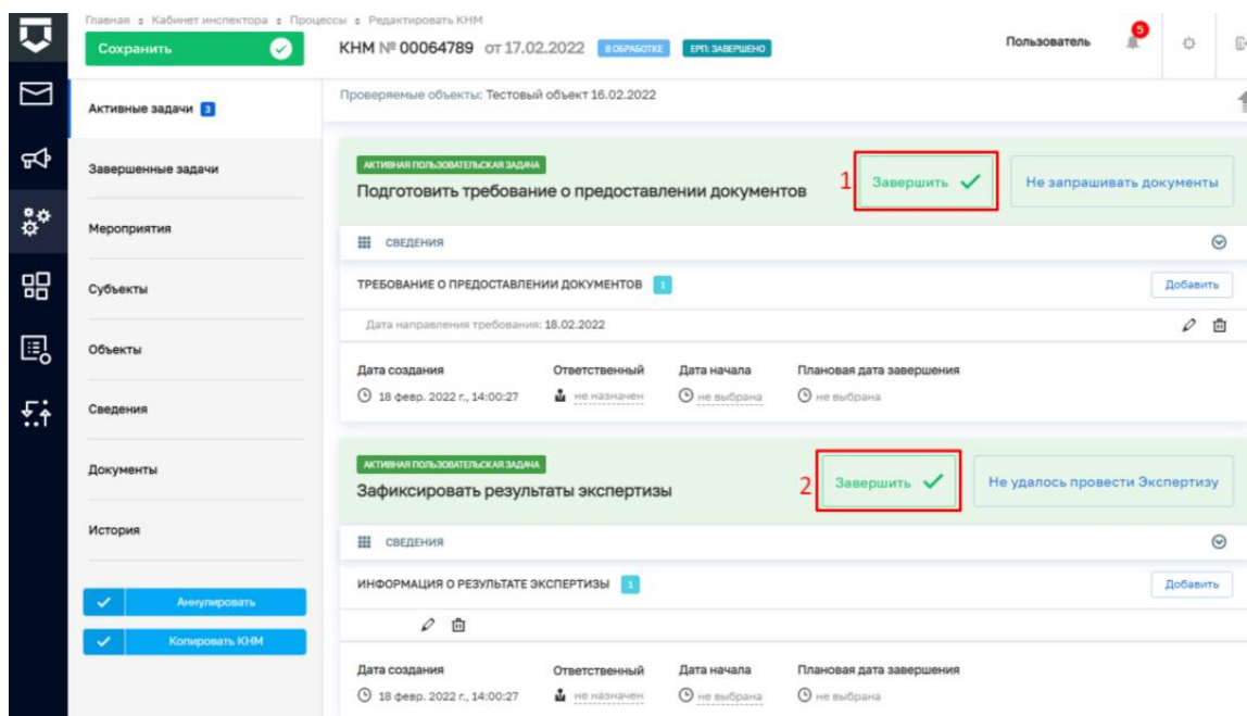
Рисунок 25. Завершение работы с задачами "Подготовить требование о предоставлении документов" и "Зафиксировать результаты экспертизы"
